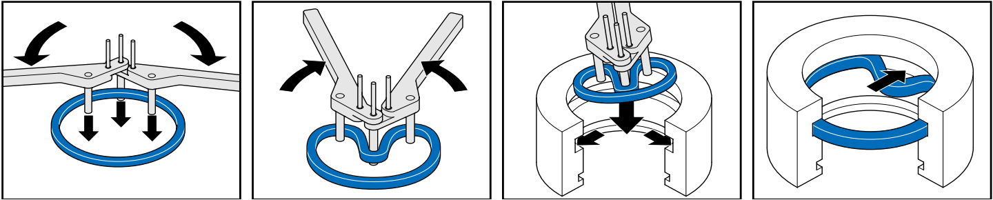
1A. 通过夹钳进行安装
