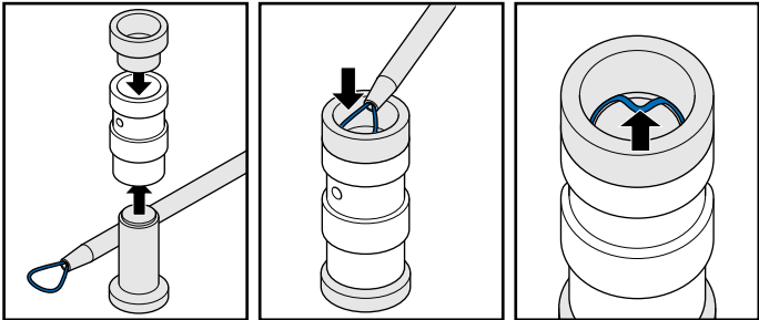
2. O形圈安装
