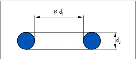
符合ISO 3601的设计
