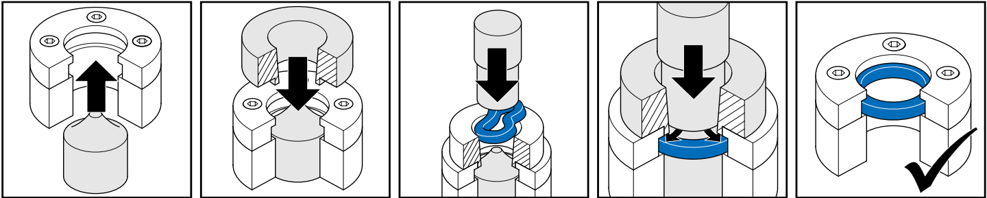
1B. 通过工装安装
